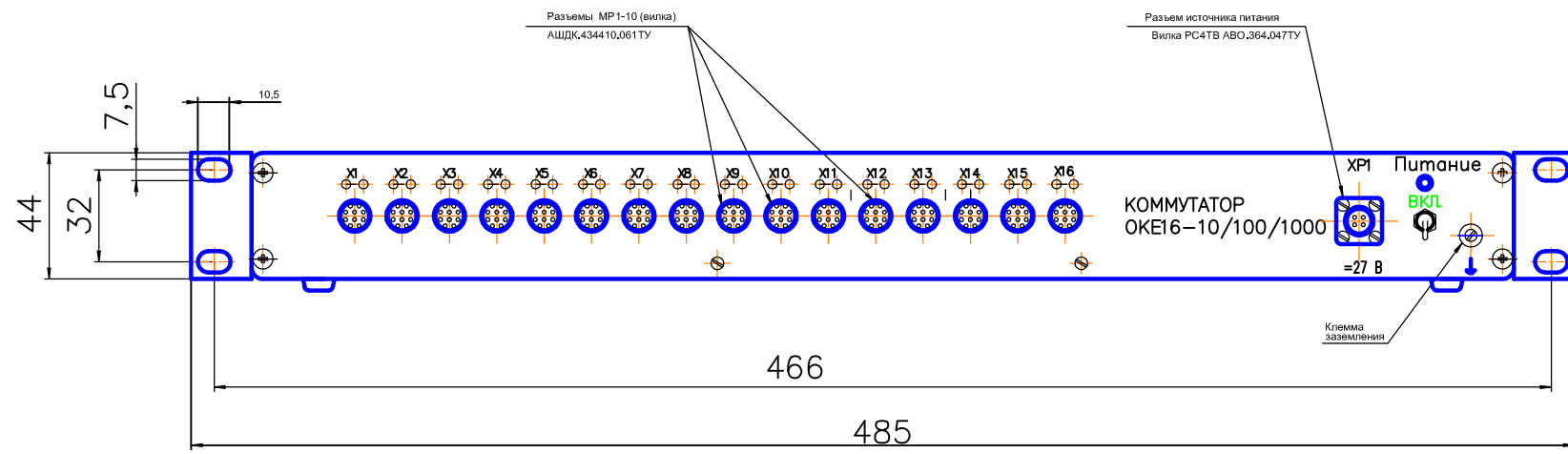
Коммутатор ОКЕ 16-10/100/1000 ЯИМП.468352.018-02 Общий вид
