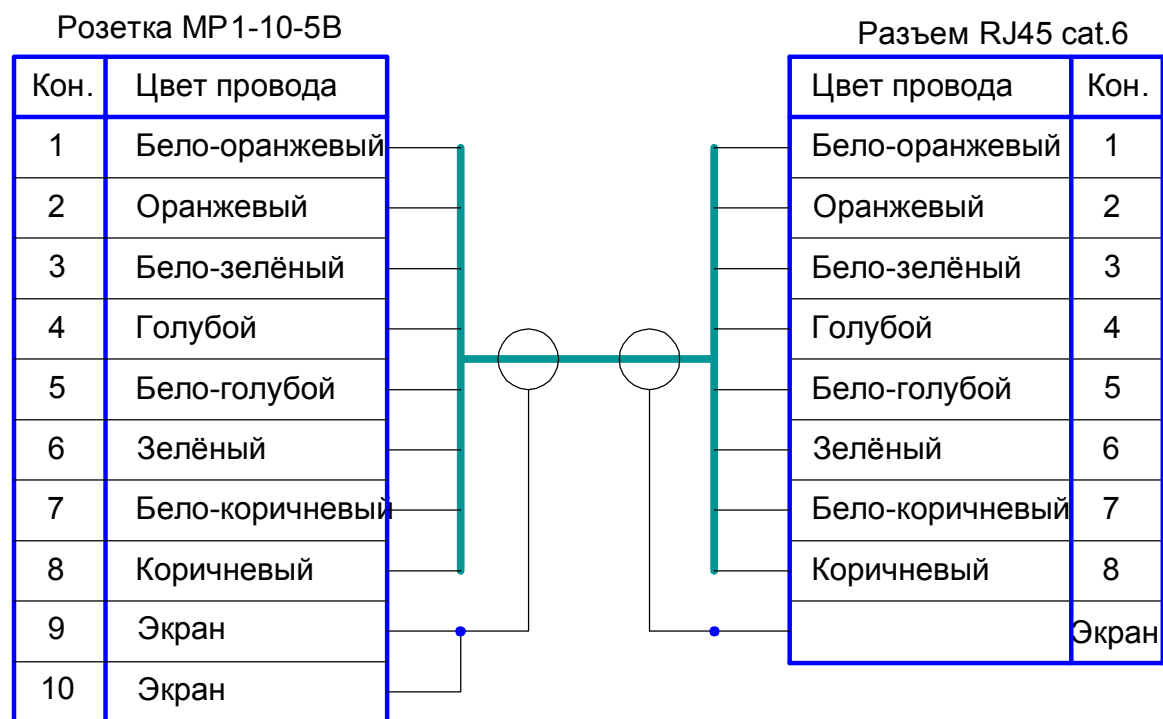
Электрическая схема соединения контактов разъемов
