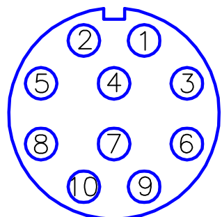
Расположение контактов розеток MP 1-10 вид со стороны пайки
